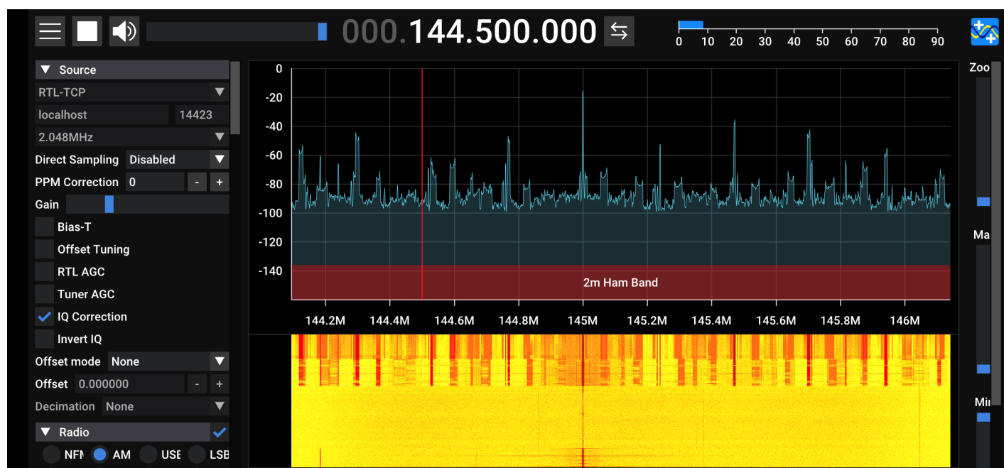
Signaal ontvangst in SDR++ zonder 20dB attenuator
